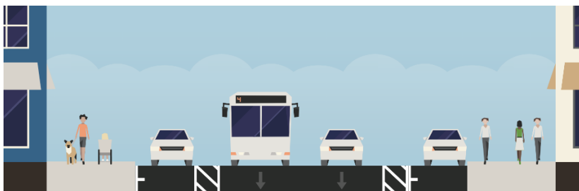
القطاع العرضي المقترح للشارع في ليفنورث (LEAVENWORTH)
