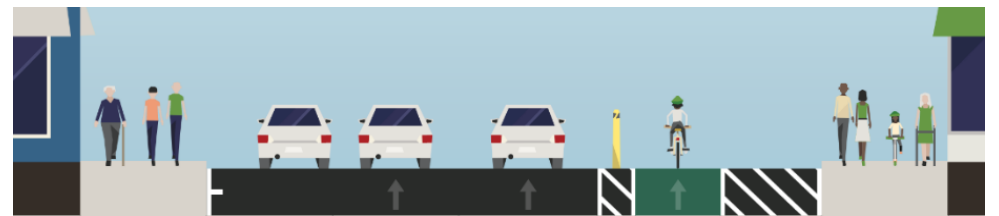
القطاع العرضي المقترح للشارع في ليفنورث (GOLDEN GATE)
