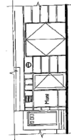
4 Muni Breakroom Elev. Scale: 1/8" = 1'-0"
